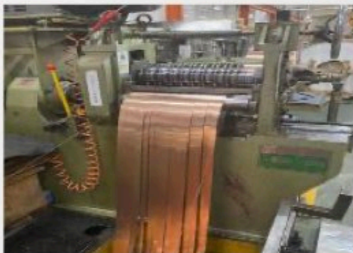
分条设备
